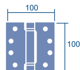
Bisagra simple acción 100mm Referencia: N1040 Código: 21104
