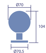
Pomo bola puerta entrada SOBREPONER Referencia: PE/70SOB-INOX Código: 26936
