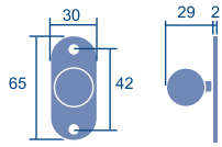
Tirador maletero Referencia: I018 Código: 25946 20 udes.
