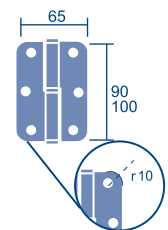
Bisagra quita y pon canto redondo
