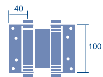
Bisagra doble acción 100mm Referencia: N222/100inox Código: 23239
