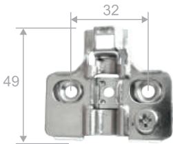
Base regulación excéntrica H0 y H2
