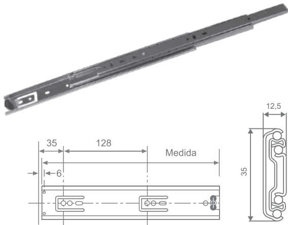
Juego guía con rodamientos extracción total H35.
