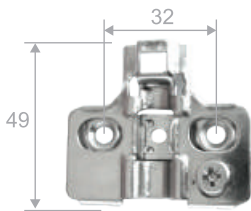
Base regulación excéntrica H0 y H2
